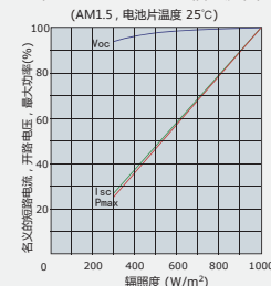
Isc, Voc and Pmax的辐照度曲线
