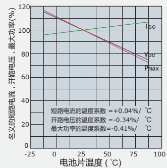
Isc, Voc and Pmax的温度曲线
