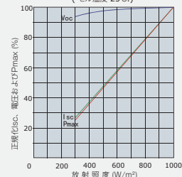
Isc, VocとPmaxの放射照度依存性 (セル温度 25°C)
